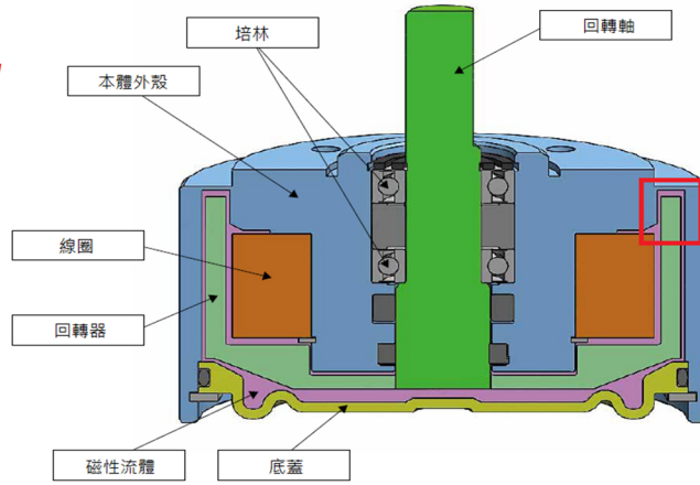
電控緩衝器的構造如下圖所示
