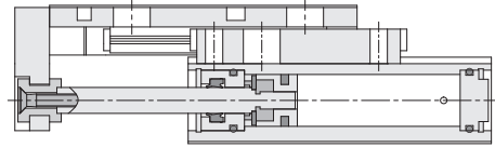
◎ 內部結構圖
