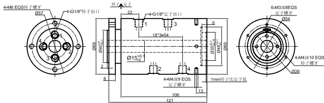
GJ4015-02 尺寸图 4进4出, G1/8接头
