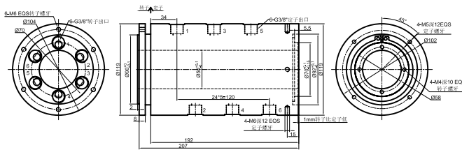
GJ6050-04 尺寸图 6进6出, G3/8接头
