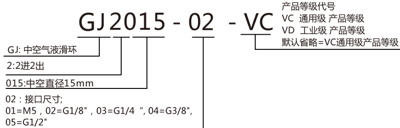
GJ2015-02 尺寸图 2进2出, G1/8接头
