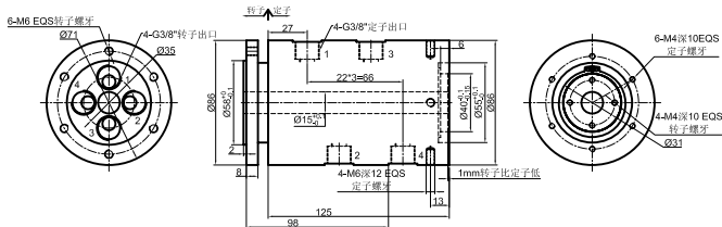
GJ4015-04 尺寸图 4进4出, G3/8接头
