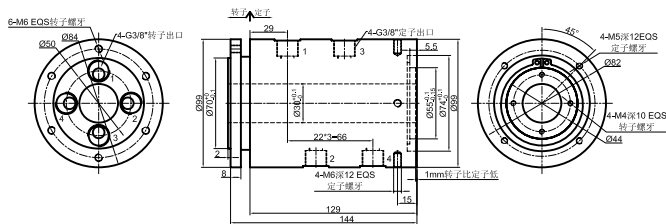
GJ4030-04 尺寸图 4进4出, G3/8接头
