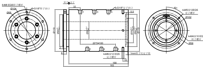
GJ6050-02 尺寸图 6进6出, G1/8接头
