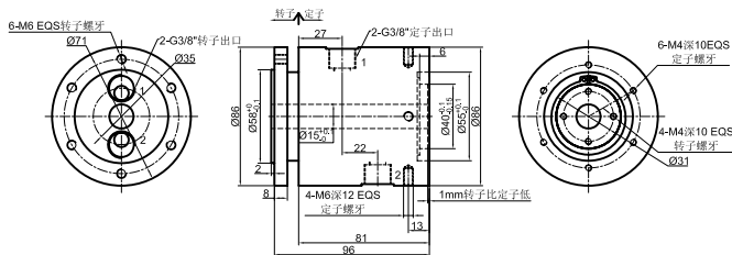
GJ2015-04 尺寸图 2进2出, G3/8接头
