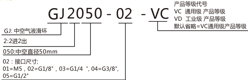
GJ2050-02 尺寸图 2进2出, G1/8接头
