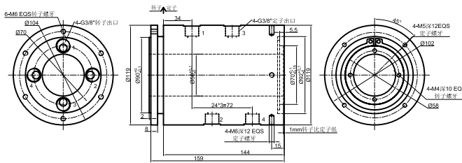
GJ4050-04 尺寸图 4进4出, G3/8接头
