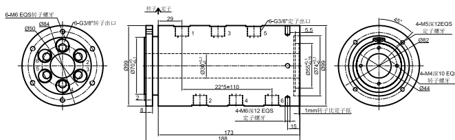
GJ6030-04 尺寸图 6进6出, G3/8接头
