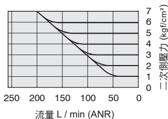
● ERX-300 洩放特性
