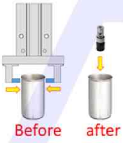
感光鼓夾取模組
